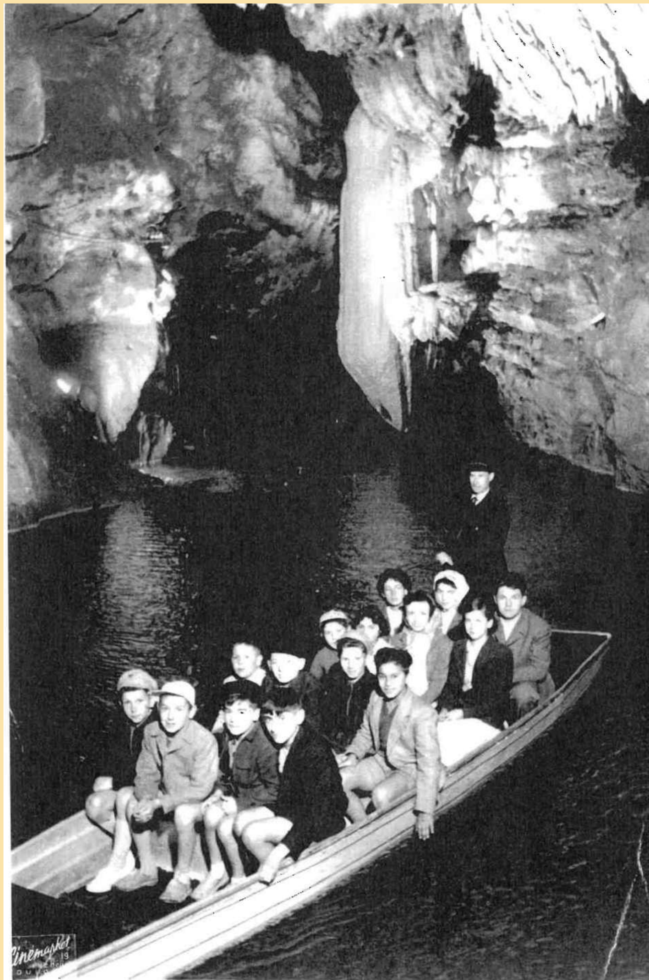
LUFFRE DE PADIRAC - Le lac de la Pluie
