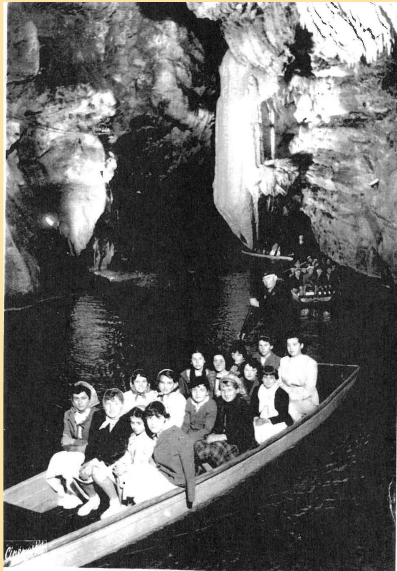
GOUFFRE DE PADIRAC. Le lac de la Pluie.
